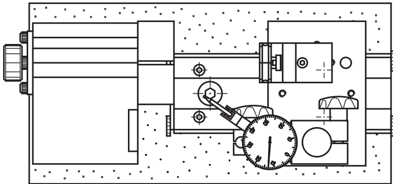
Beispiel mit Prisma als Gegenlager für lange Teile
